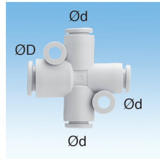
Křížová spojka, tři redukováané vývody KQ2TY
