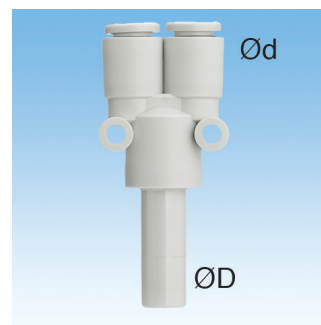
U-spojka s čepem, redukovaná KQ2X
