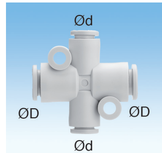
Křížová spojka, dva redukováané vývody KQ2TX
